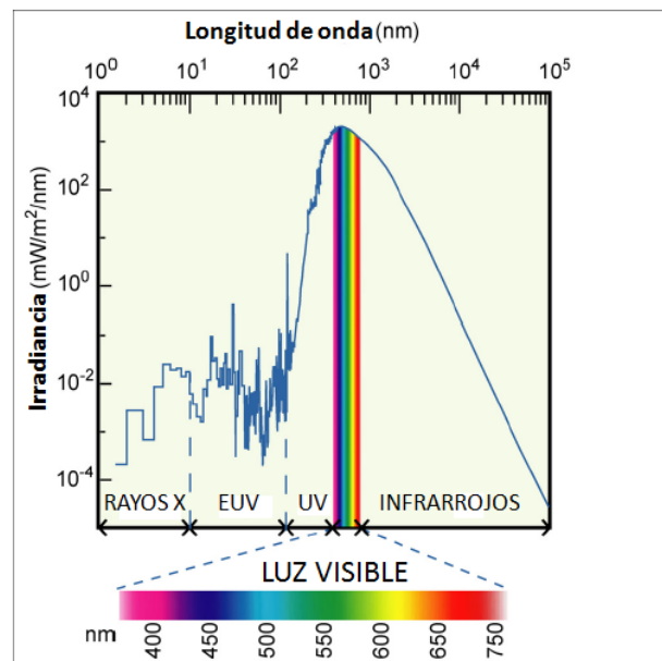
Figura 24. Irradiancia solar desde 1 nm hasta 100 \mu m, con la región visible del espectro (380-750 nm) resaltada. EUV: Ultravioleta extremo. UV: ultravioleta (Purcell y Crosson 2008)
