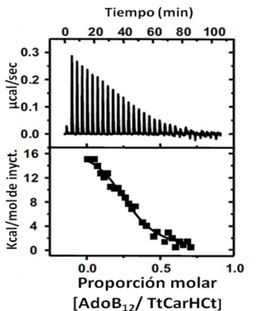
Figura 57. ITC con 18 \mu\text{M} de TtCarHCt titulado con 78 \mu\text{M} de AdoB 12 a 25 °C. Panel superior: cambio de calor con cada inyección. Panel inferior: Calor integrado normalizado y corregido para el calor de la dilución frente a la proporción molar. La línea que mejor se ajusta a los datos corresponde con el modelo de un único sitio de unión.
