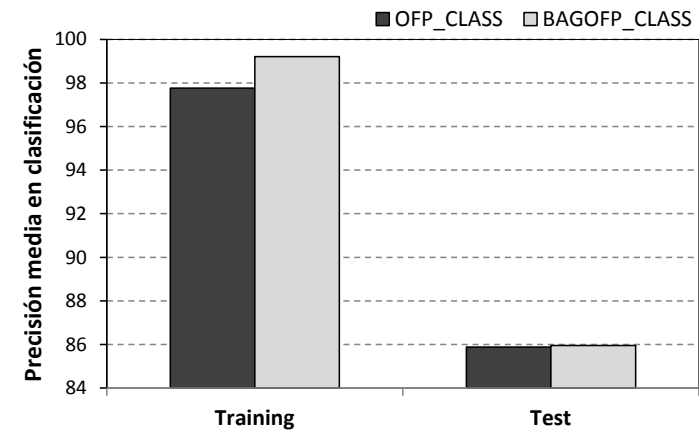
Figura 10.12: Comparando los resultados de los conjuntos de datos que verifican |E| \geq 10 \cdot |A| \cdot |C|
