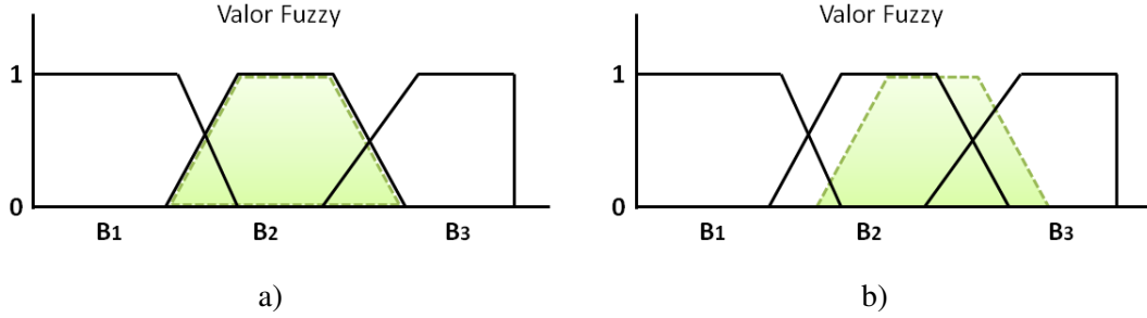
Figura 6.5: Manejo de los valores fuzzy en el FDT a) y en el ensamble FDT LQD b)
